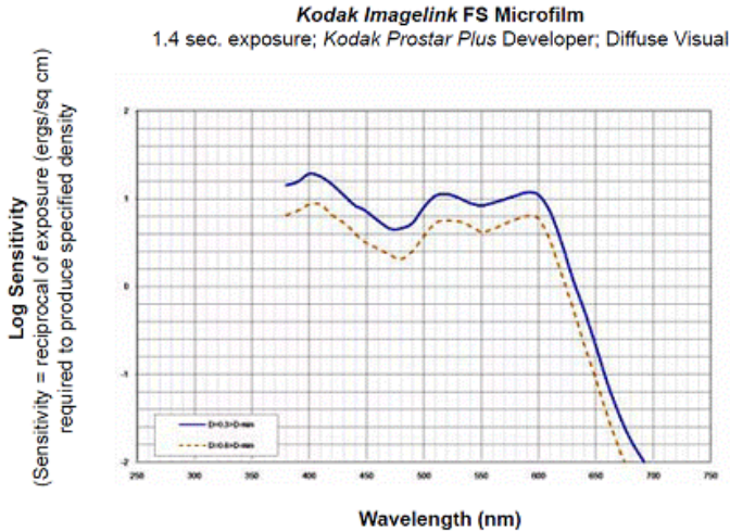
Рисунок 3 – Характеристическая кривая и кривая спектральной чувствительности фотопленки «Imagelink HQ 1461/2461/3461 Microfilms FS 1455/3455 Microfilms UC 3454 Microfilm D-30»
