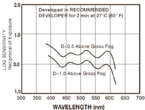
Рисунок 2 – Характеристическая кривая и кривая спектральной чувствительности фотопленки «FUJIFILM MICROFILM NEGATIVE HR11»
